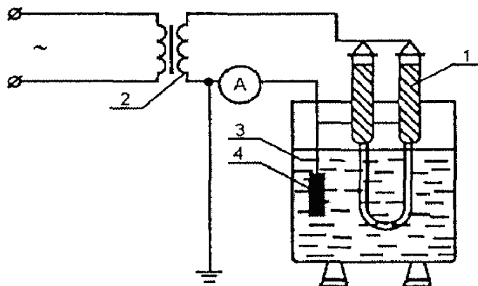
Рис. 2.1. Принципиальная схема испытания электрической прочности изоляции рукояток и провода указателя напряжения:
