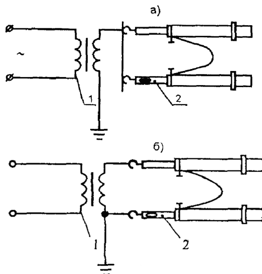
Рис. 2.2. Принципиальные схемы испытания указателя напряжения для проверки совпадения фаз по схеме согласного (а) и встречного (б) включения:
